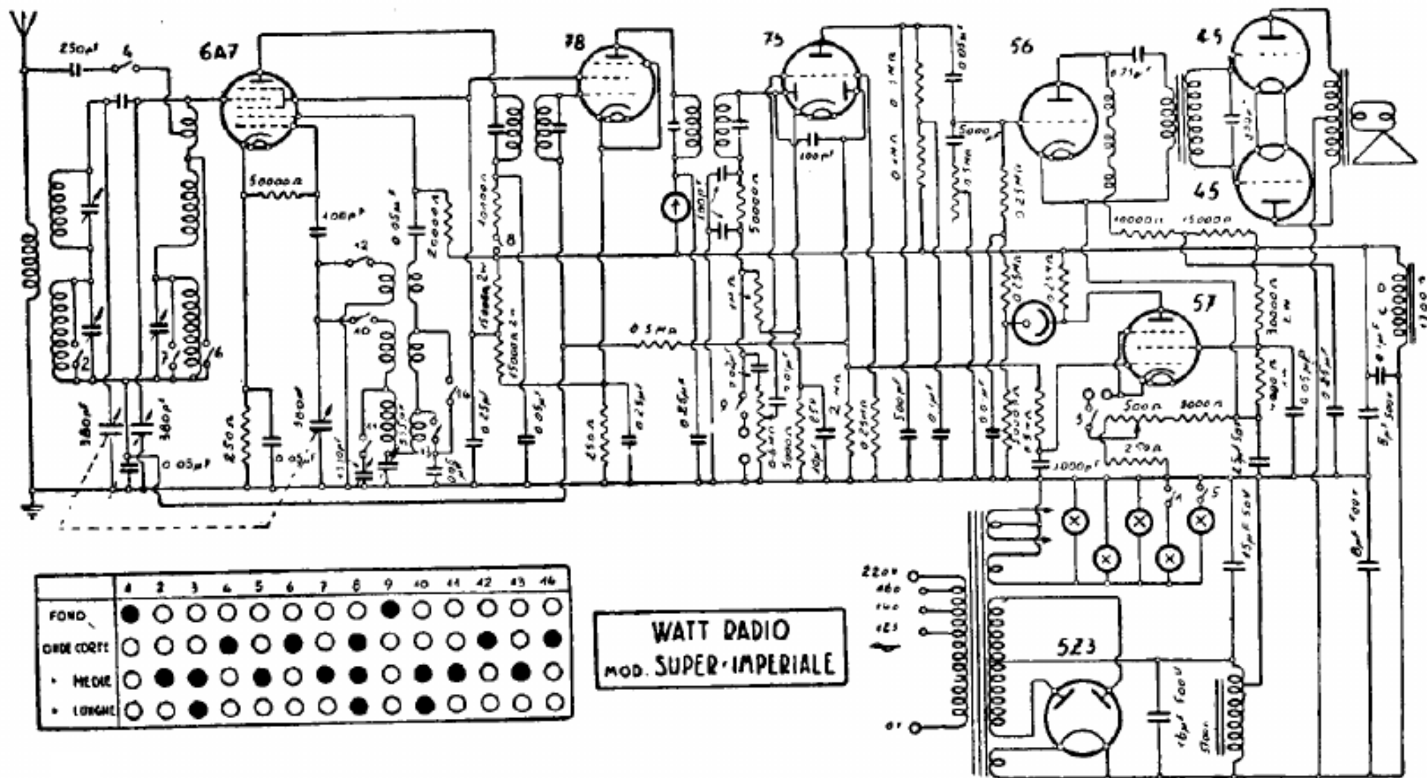
WATT RADIO — Mod « Super Imperiale » · Produzione 1937.
